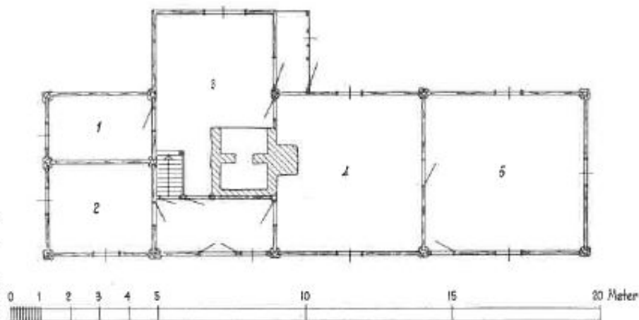
Bild 175. Signe Gunnarssons gård, Blixtorp, Årstad, plan.
